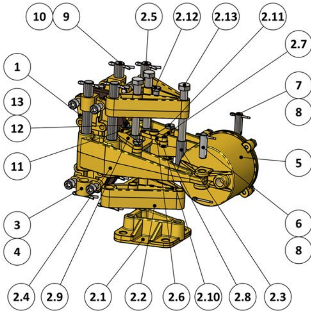
5019-A Caliper Brake
