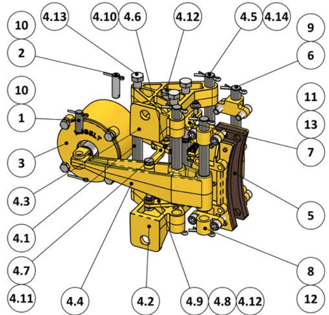
5019-AW Caliper Brake
