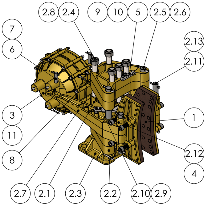
5024-A Caliper Brake
