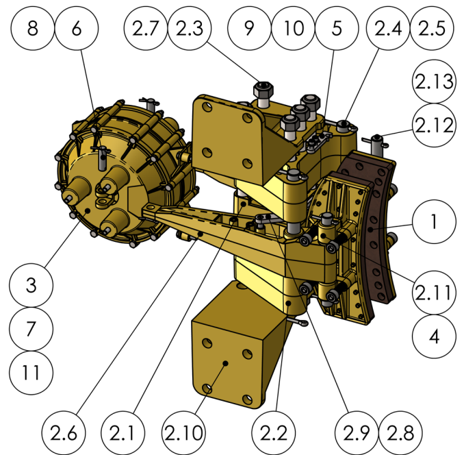
5024-AW Caliper Brake
