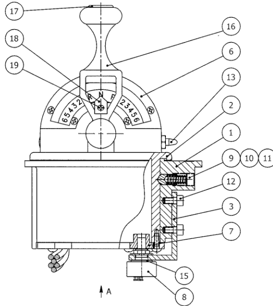
VIEW A-A
