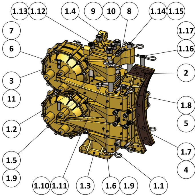
5027-A Caliper Brake
